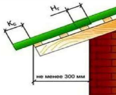
Рис. 1 Карниз кровли
