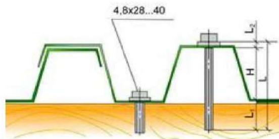
Рис. 2 Крепление листов профнастила
