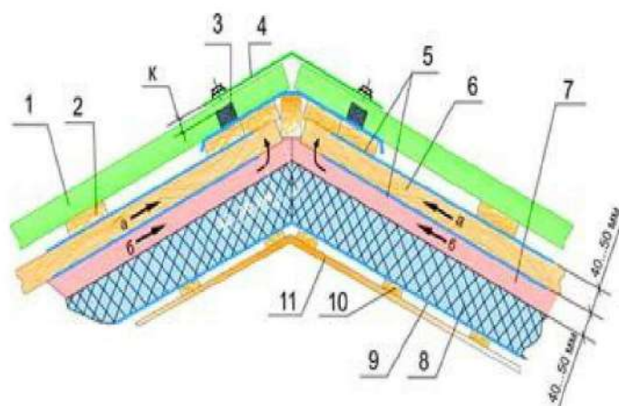
Рис.5 Утепление кровли
