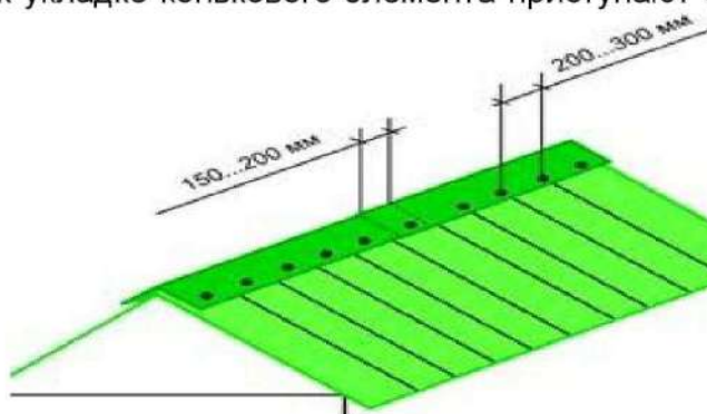
Рис. 10 Крепление конькового элемента
